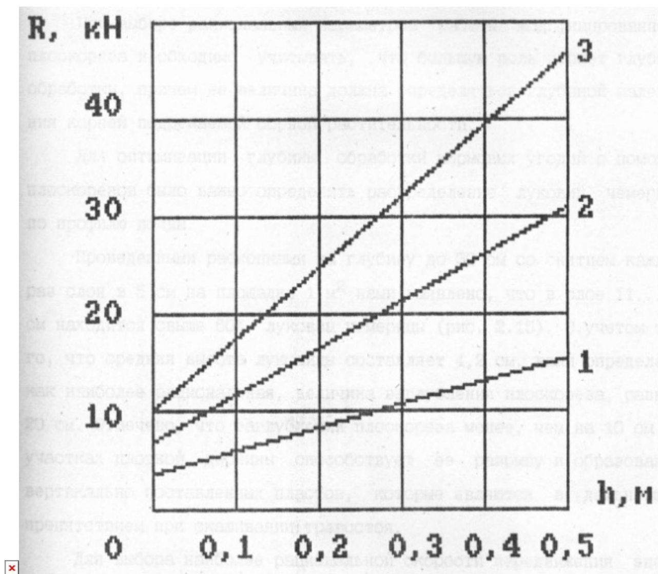
Рис. 4. Зависимость удельного сопротивления плоскорезного агрегата от глубины обработки почвы при работе на IV передаче с одним (1), двумя (2) и тремя (3) рабочими органами.
