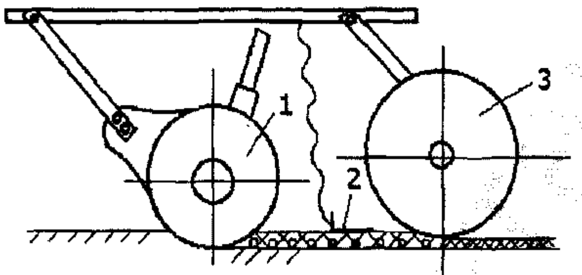
Рис. 3. Схема технологического процесса сеялок с прикатывающими катками
