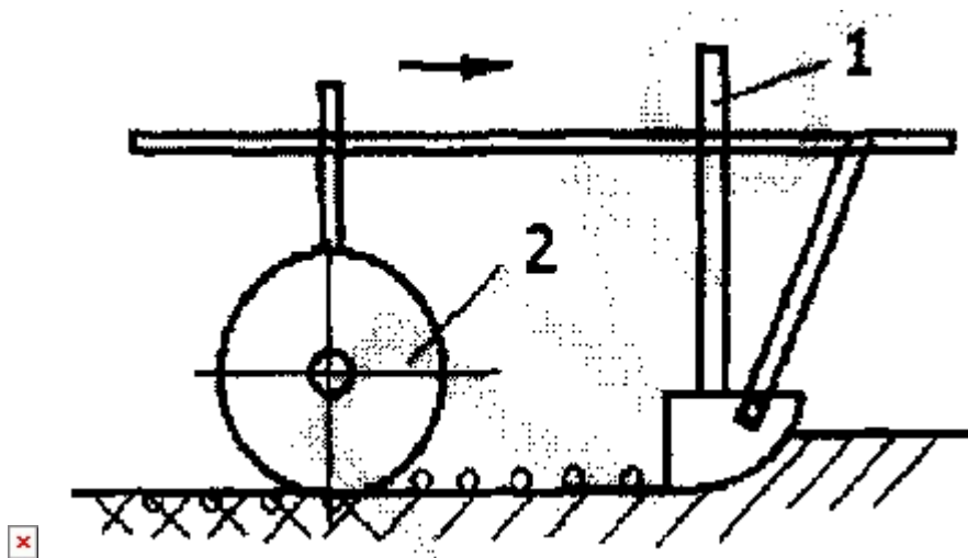
Рис. 4. Комбинированный сошник конструкции А.И. Беднова
