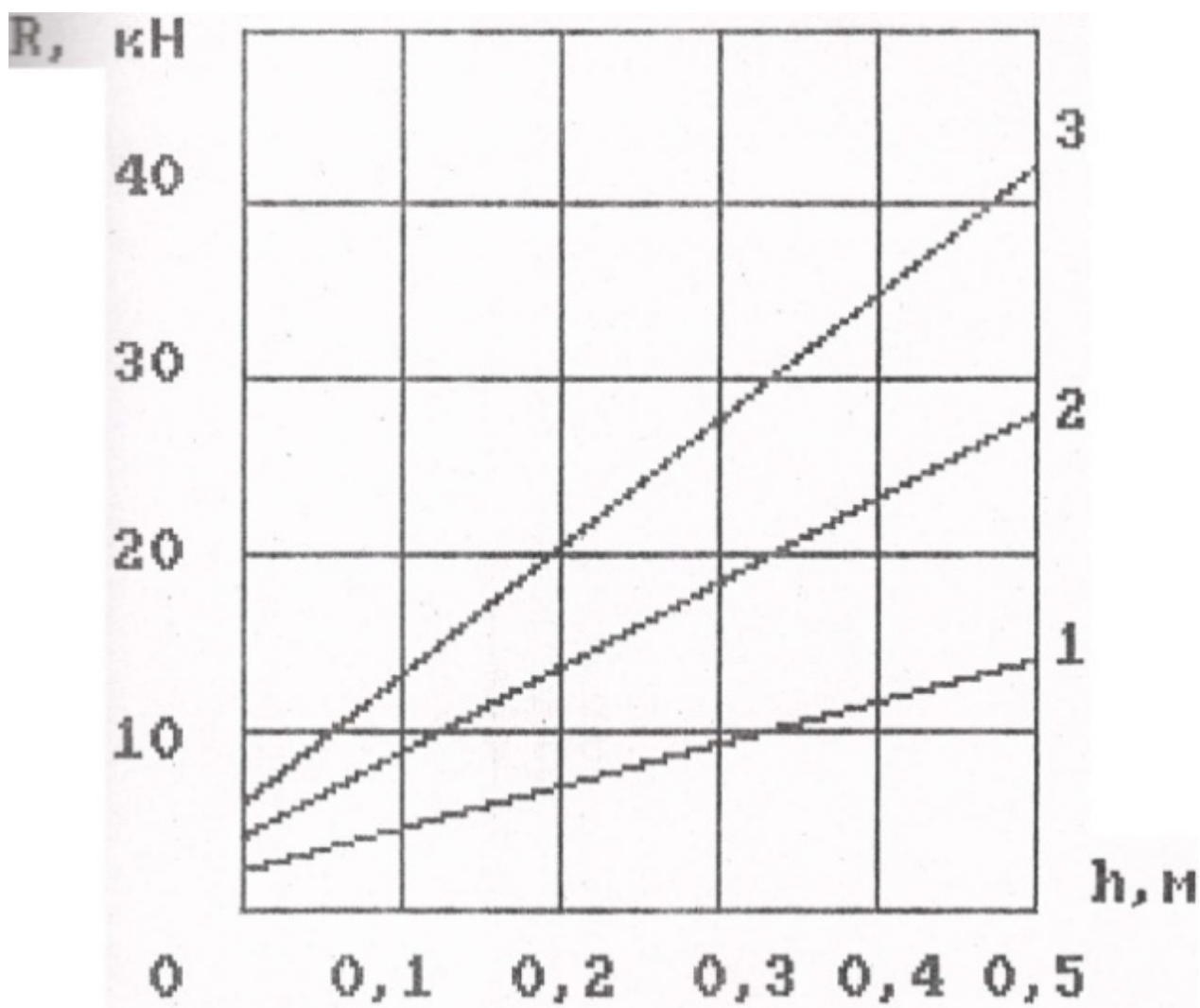
Рис. 2. Зависимость удельного сопротивления плоскорезного агрегата от глубины обработки почвы при работе на II передаче с одним (1), двумя (2) и тремя (3) рабочими органами.
