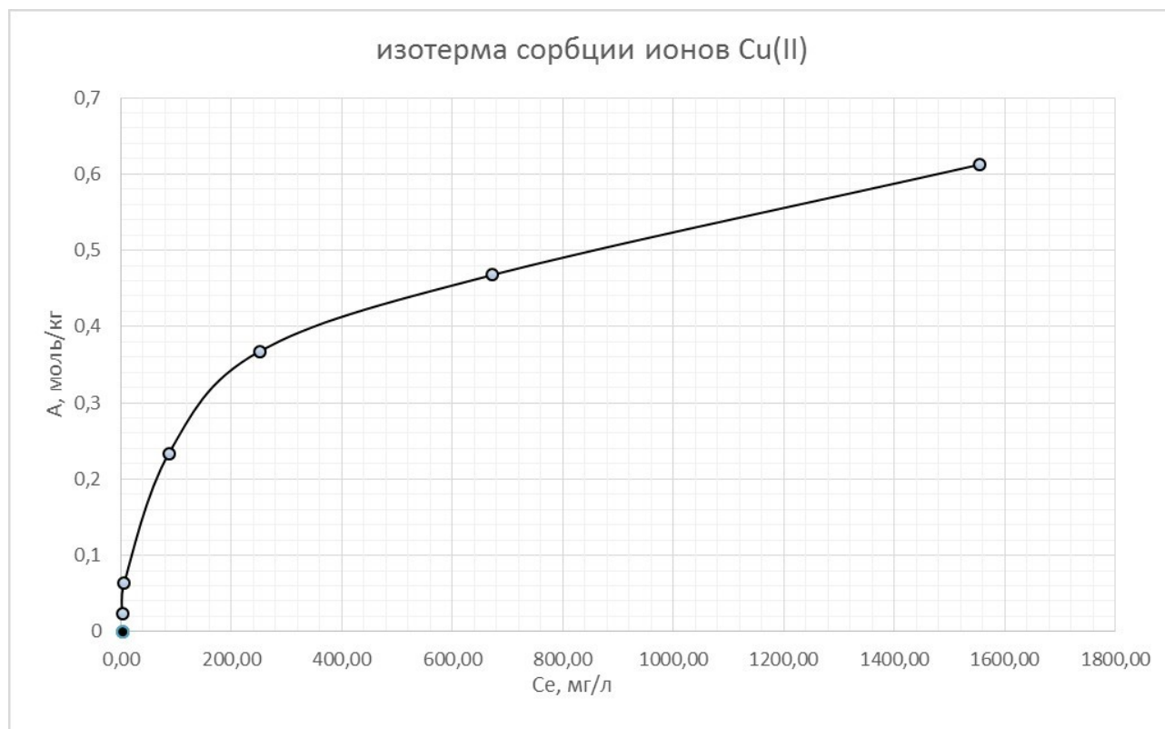
Рис.4. Изотерма сорбции ионов меди (II)
