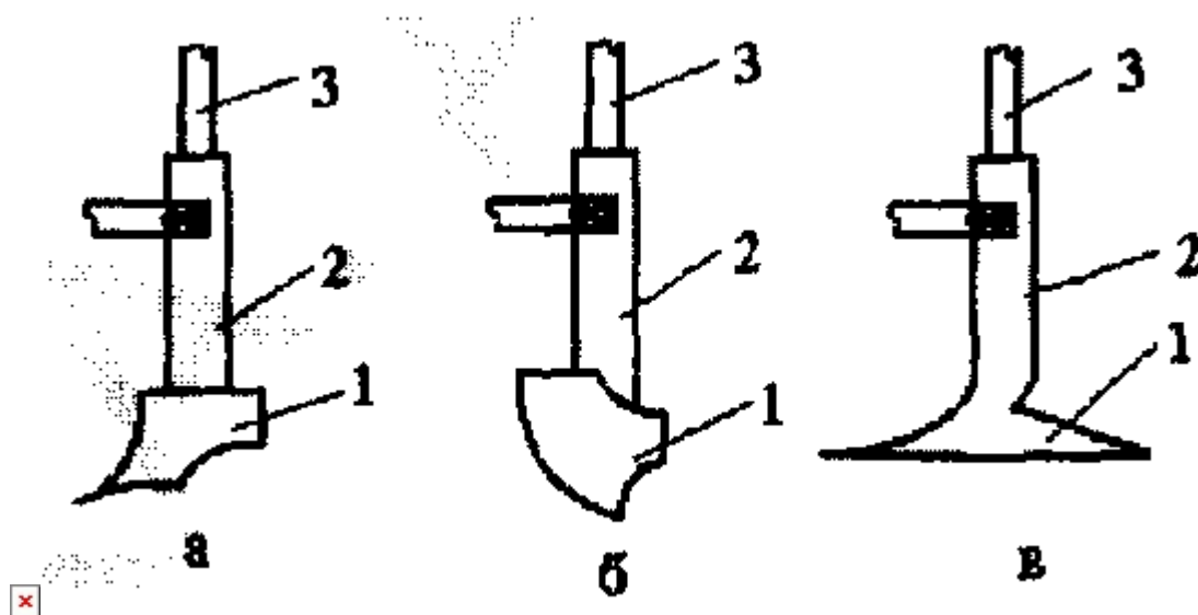
Рис. 2. Наральниковые сошники: а – анкерный; б – килевидный; в – в виде стрелчатой лапы
