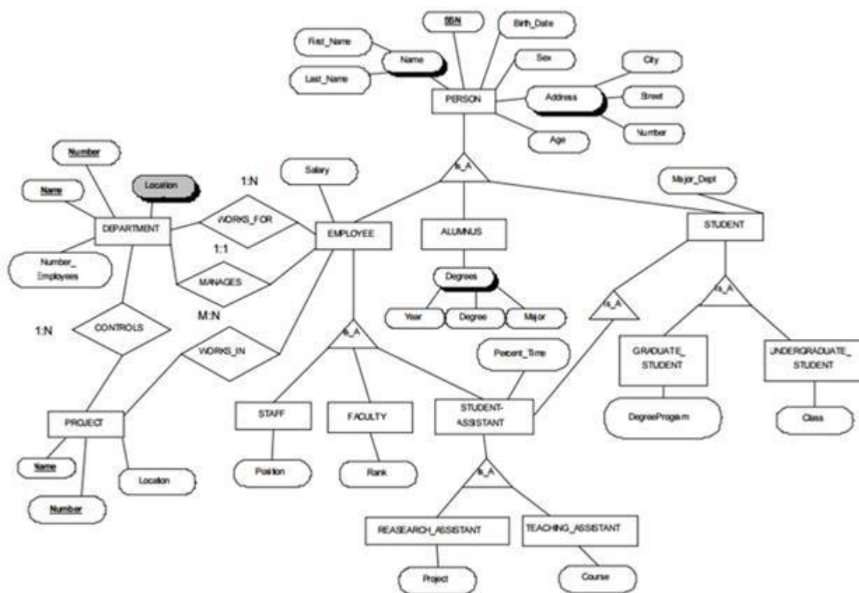
Рис. 2. Пример диаграммы №2 в нотации Чена
