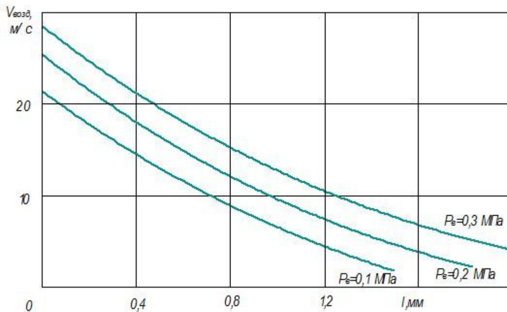
Рисунок 4 – Зависимость скорости движения воздуха V_{\text{в}} от l и P_{\text{в}} при оптимальной высоте воздушного сопла h=0,2 мм
