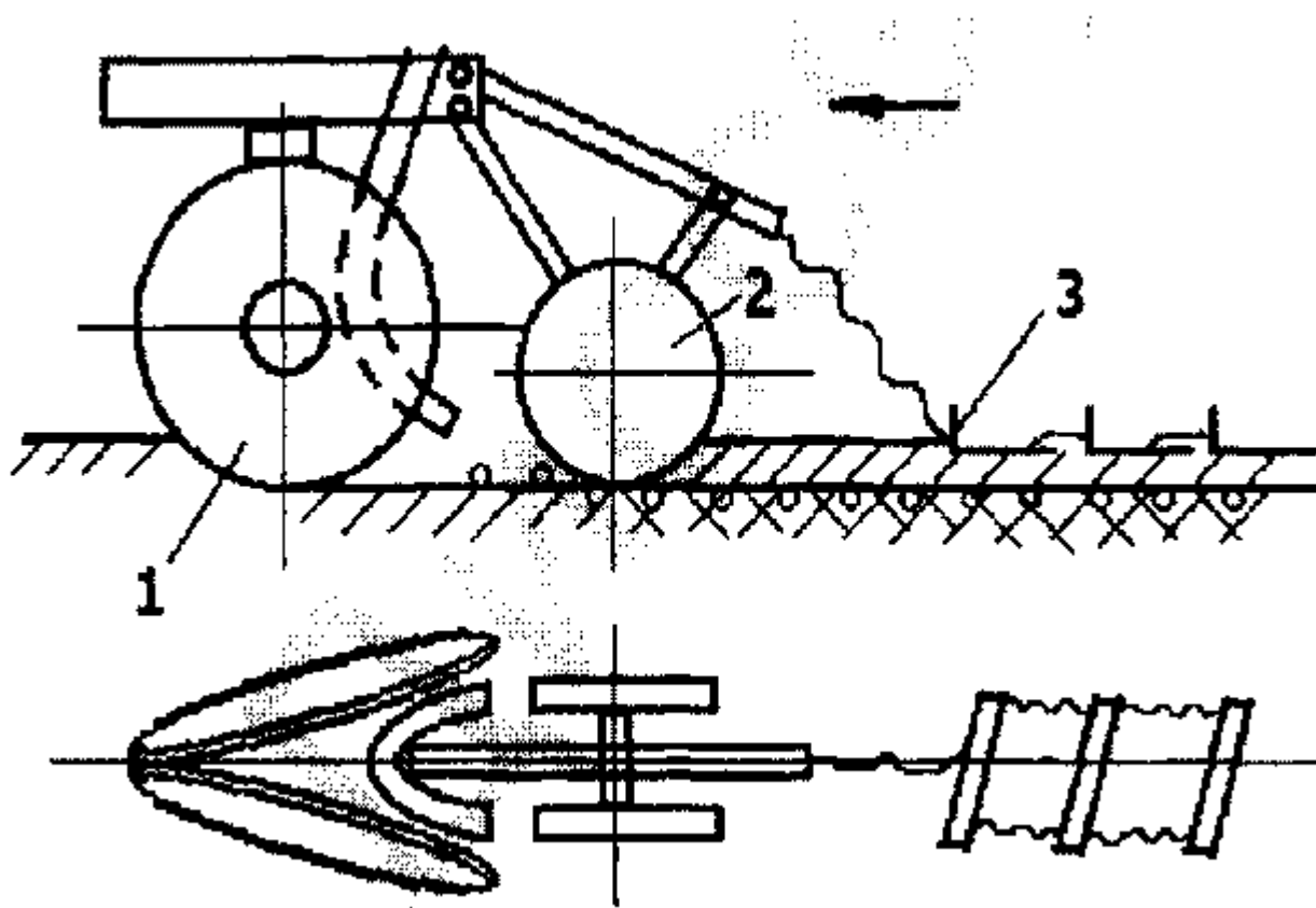
Рис. 5. Комбинированный сошник Х.С. Гайнанова
