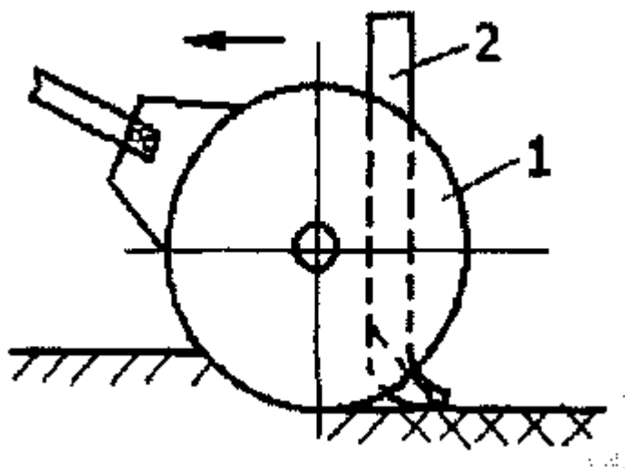
Рис. 7. Сошник Ф.Е. Аниферова
