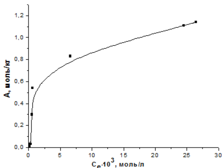
Рис. 2 – Изотерма сорбции ионов Cu(II) сорбентом из стеблей топинамбура
