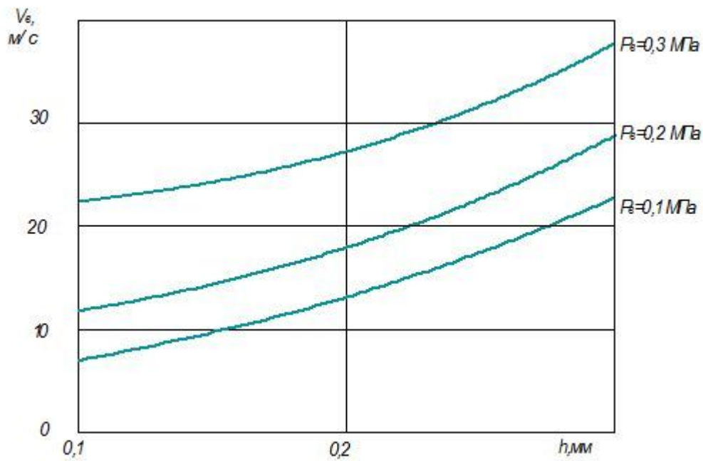
Рисунок 2 – Зависимость скорости движения воздуха V_{\text{в}} от P_{\text{в}} и высоты h щелевого сопла на расстоянии от него 0,35 мм.
