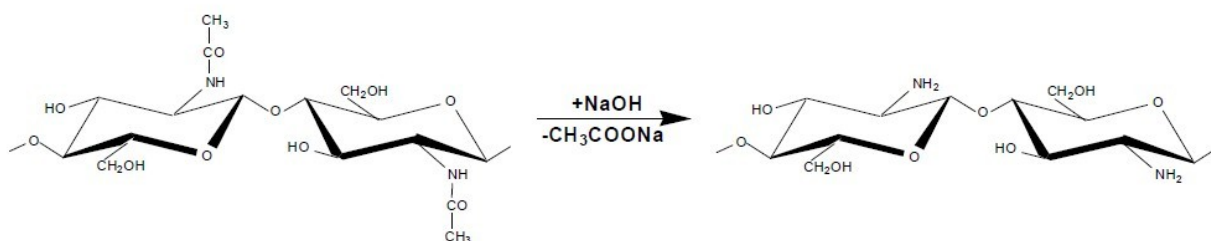
Рис.1. Схема получения хитозана из хитина
