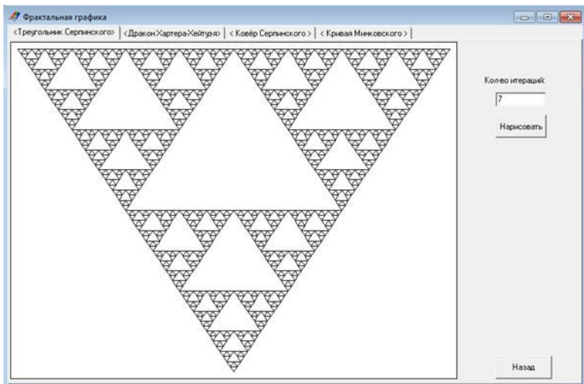
Рис. 2 Треугольник Серпинского
