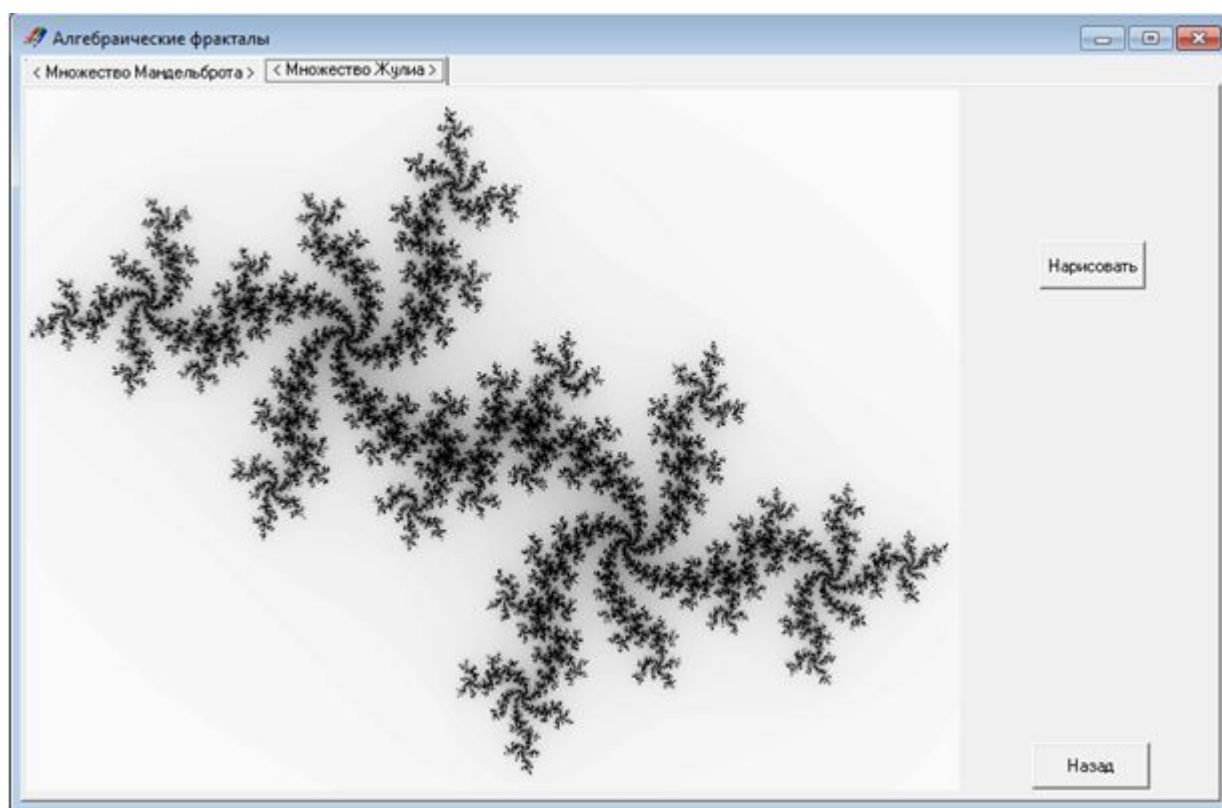
Рис. 3 Множество Жулиа
