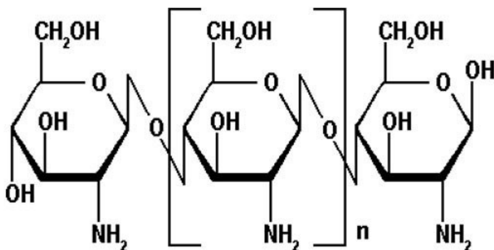
Рис. 2. Структурная форма хитозана
