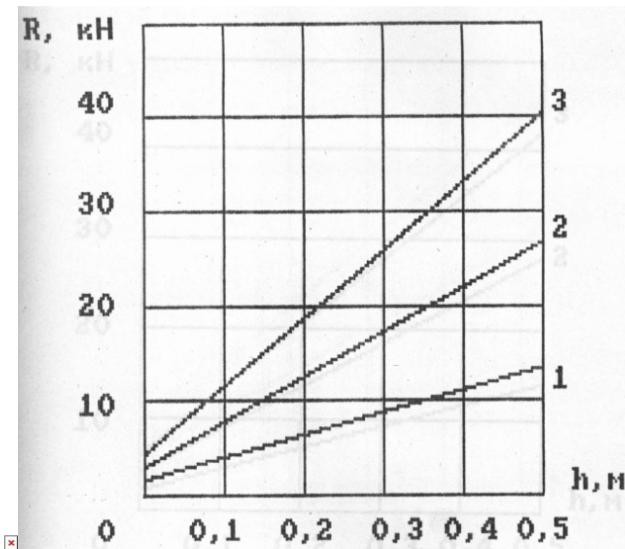
Рис. 1. Зависимость удельного сопротивления плоскорезного агрегата от глубины обработки почвы при работе на I передаче с одним (1), двумя (2) и тремя (3) рабочими органами.
