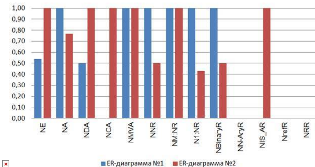
Рис. 3. Нормированные значения количественных метрик ER-диаграмм
