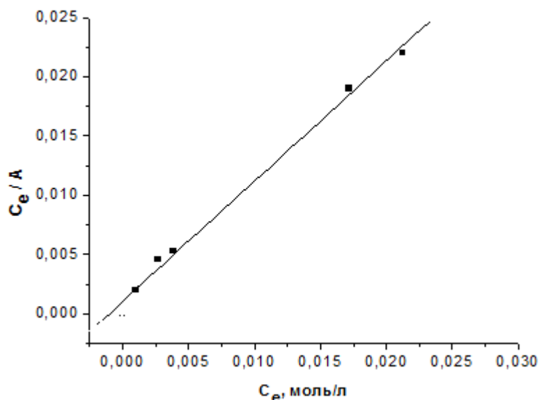
Рис. 3 – Обработка изотермы сорбции ионов Cu(II) по модели Ленгмюра
