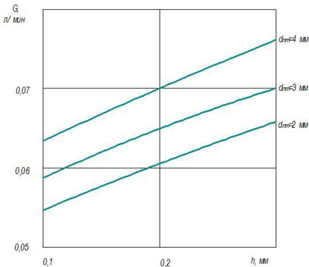
Рисунок 1 – Зависимость расхода жидкости G от h и d_{пт} при оптимальном давлении воздуха P_v=0,2 МПа.
