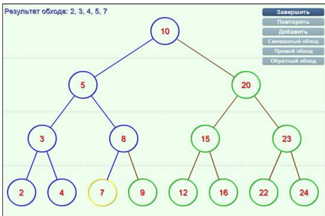
Рис. 3. Демонстрация алгоритма обхода
