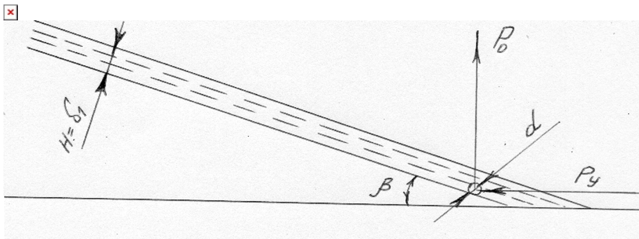
Рисунок 1 – Схема для расчета сопротивления почвы смыву
