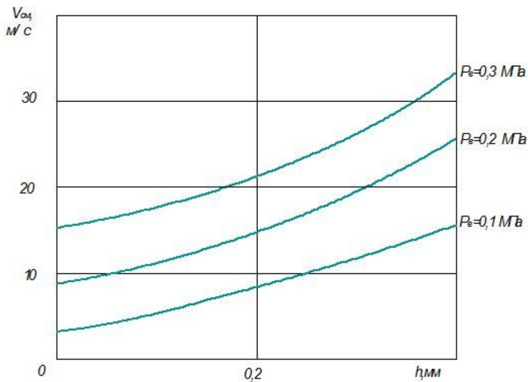
Рисунок 3 – Зависимость скорости движения воздушно – капельной смеси V_{\text{см}} от P_{\text{в}} и h при расстоянии от сопла 0,35 м.
