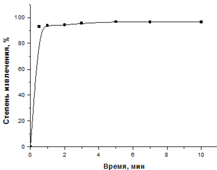
Рис. 1 – Кинетическая кривая сорбции ионов Cu(II) сорбентом из стеблей топинамбура
