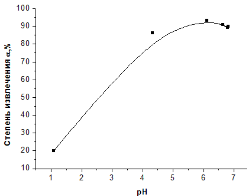
Рис. 4. Влияние pH раствора на сорбцию ионов Cu(II) сорбентом из стеблей топинамбура
