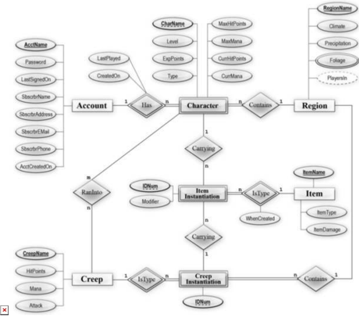
Рис. 1. Пример диаграммы №1 в нотации Чена Метрические характеристики для представленного примера ER-диаграммы в нотации Чена (рис. 1) приведены в таблице 2.
