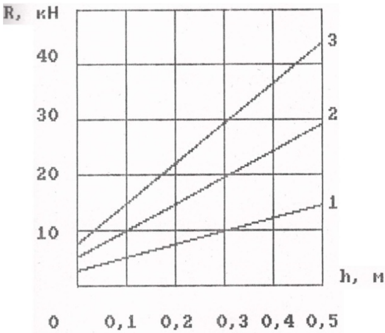
Рис. 3. Зависимость удельного сопротивления плоскорезного агрегата от глубины обработки почвы при работе на III передаче с одним (1), двумя (2) и тремя (3) рабочими органами.
