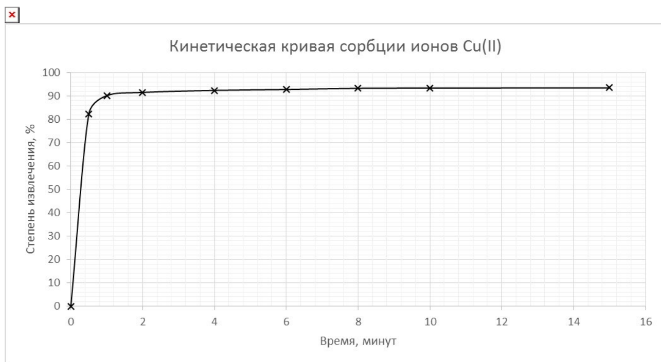
Рисунок 3. Кинетическая кривая сорбции ионов меди (II)
