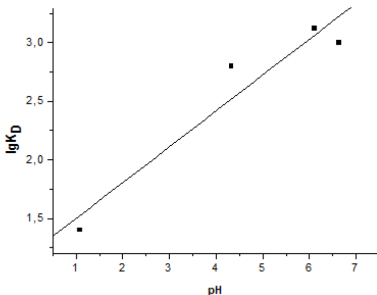
Рис. 5 – Влияние pH раствора на распределение ионов тяжелого металла в системе (\text{Me}(\text{NO}_3)_2\text{-H}_2\text{O-HNO}_3) – полисахаридный сорбент
