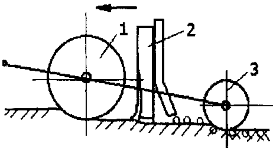
Рис. 6. Анкерно-дисковый сошник М.К. Амирханова
