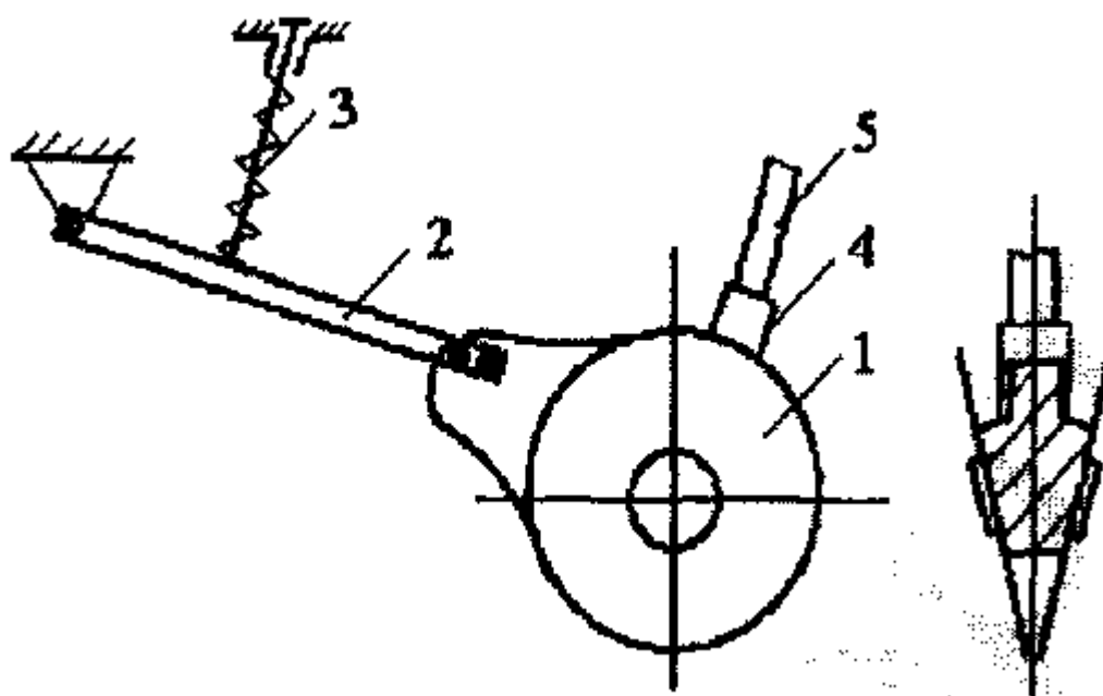
Рис. 1. Двухдисковый сошник
